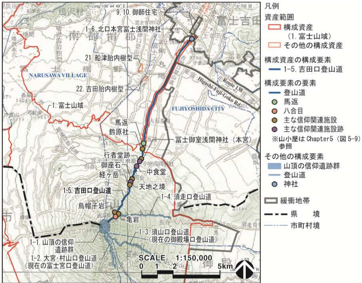
図2 吉田口登山道 平面図
