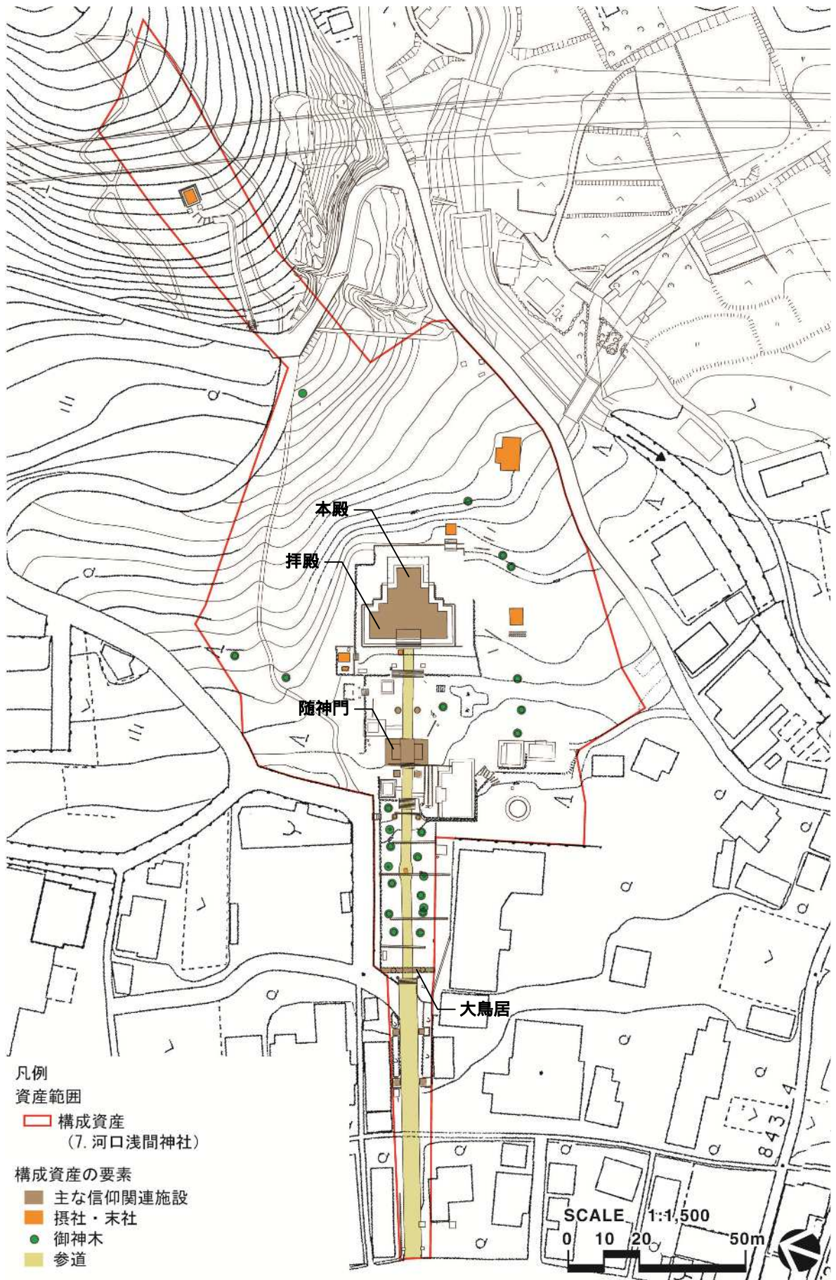
図8 河口浅間神社里宮 平面図
