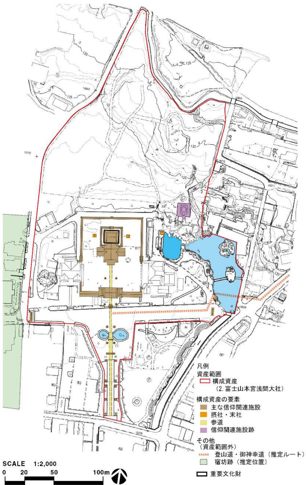
図13 富士山本宮浅間大社 平面図
